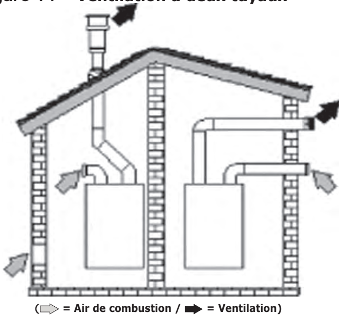
Figure 14 - Ventilation à deux tuyaux
